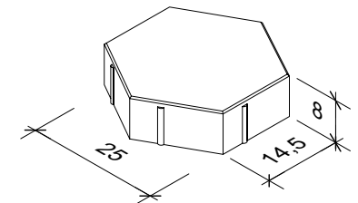
Spezialpflaster Sechskant-Vollverbund
